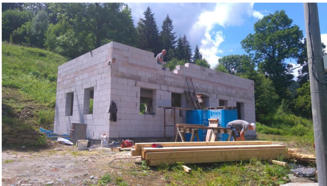
Obr.: Stavba Kutzerova domu v Horním Údolí
